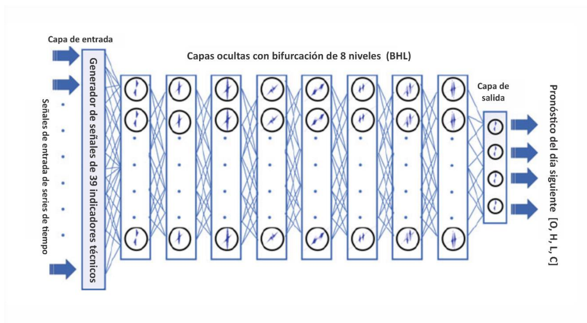
Figura 3. Arquitectura de una red neuronal profunda para minería de datos. Recuperado de “Chaotic Neural Networks in Quantum Finance” (Lee, 2020)
