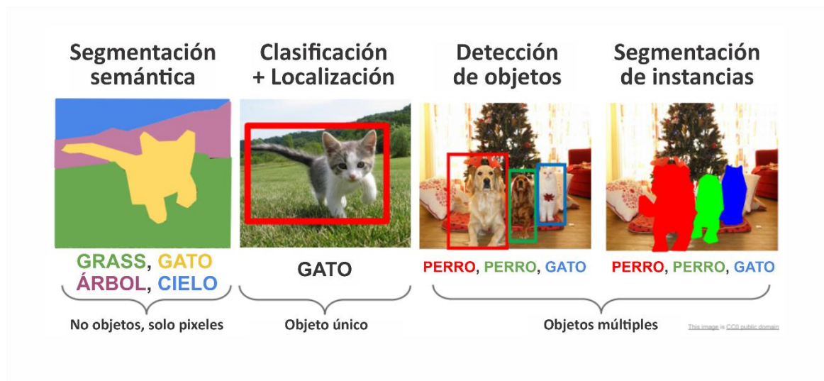
Figura 4. Tareas en visión computacional: segmentación semántica, clasificación y localización, detección de objetos, segmentación de instancias.
